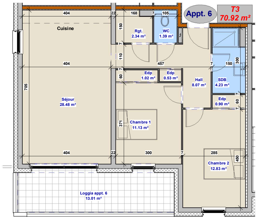
1 Appt. 6 Ech : 1 : 100
